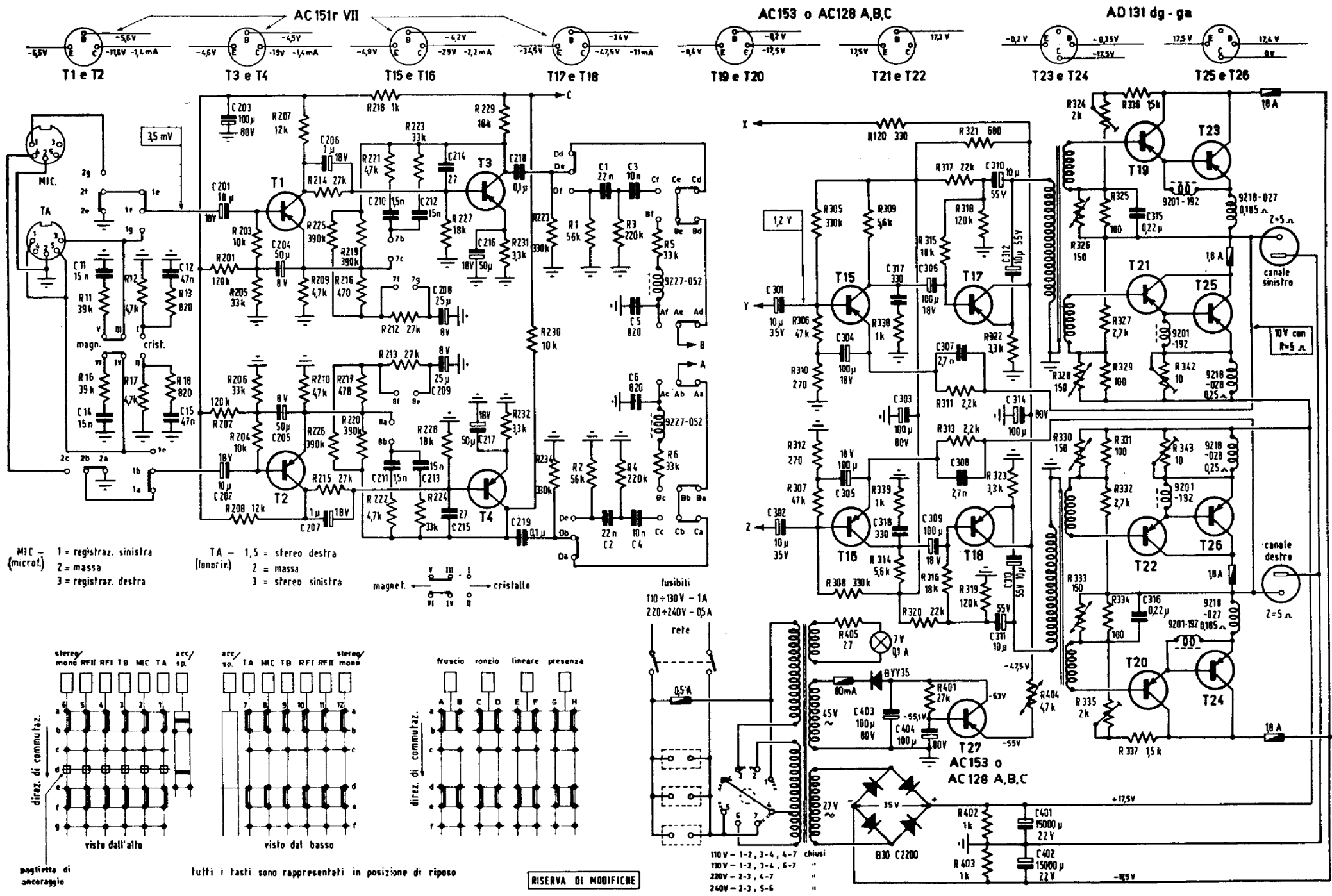
Fig. 4. - Schema elettrico dell'amplificatore stereo a transistori 2 x 20 W, SV50-Grundig.
